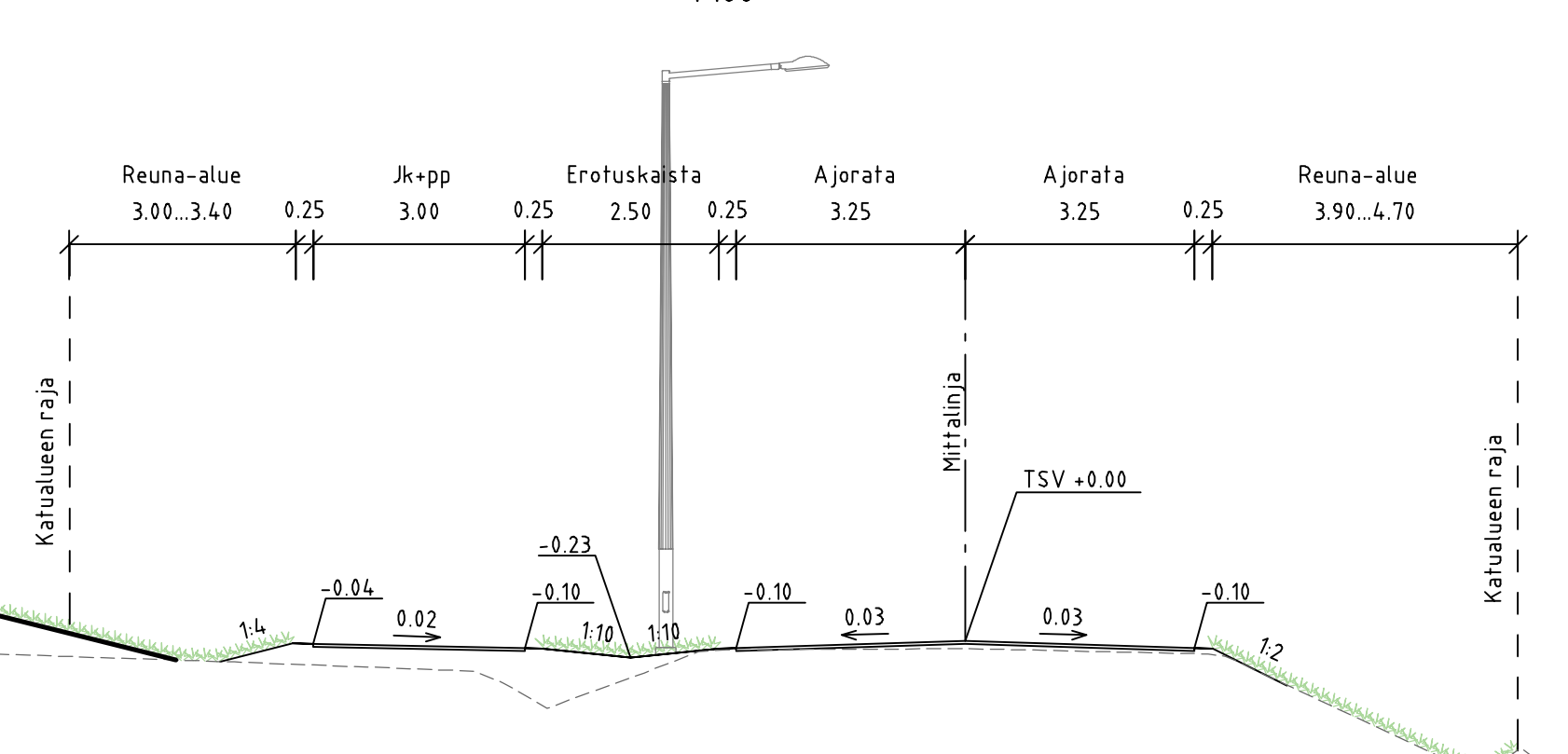
VANHATIE TYYPPIPOIKKILEIKKAUS 1:100
