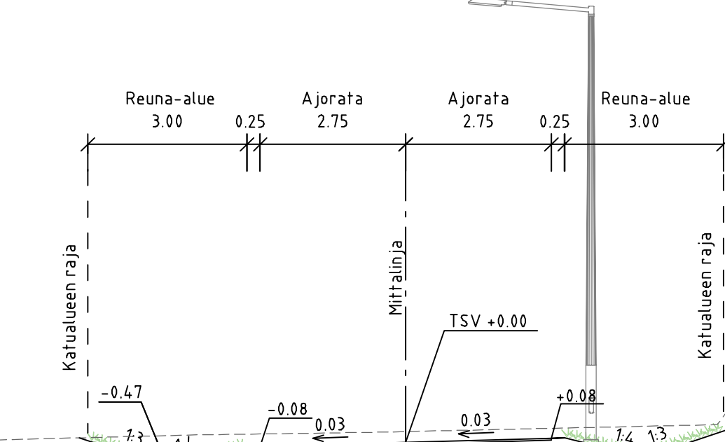
RITVANPELLOKKAARI RITVANPELLOKKAARI TYYPPIPOIKKILEIKKAUS 1:100
