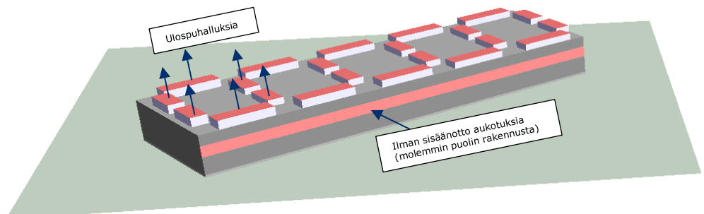
Kuva 2. Periaatteellinen kuva ilmajäähdytteisestä laitoksesta
